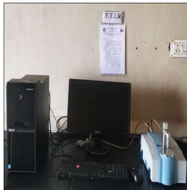
FT-IR
